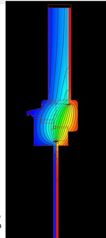
Isoterme nodo inferiore dopo
