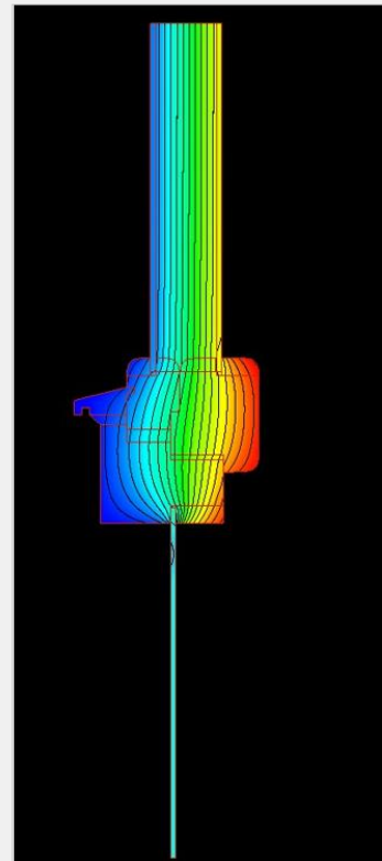
Isoterme nodo inferiore prima
